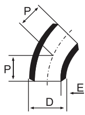
CURVA 45°
