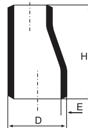
REDUÇÃO EXCÊNTRICA
