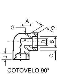
COTOVELO 90°
