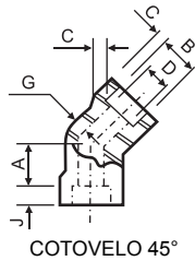
COTOVELO 45°
