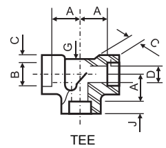
TEE
